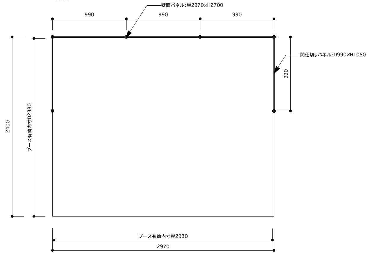
平面図 S=1:30
