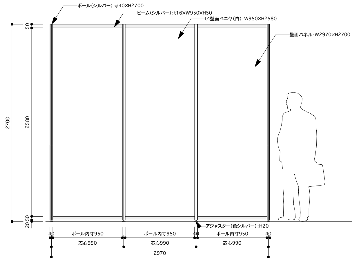
壁面立面図 S=1:30
