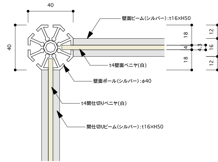
ポール・ビーム断面詳細 S=1:2
